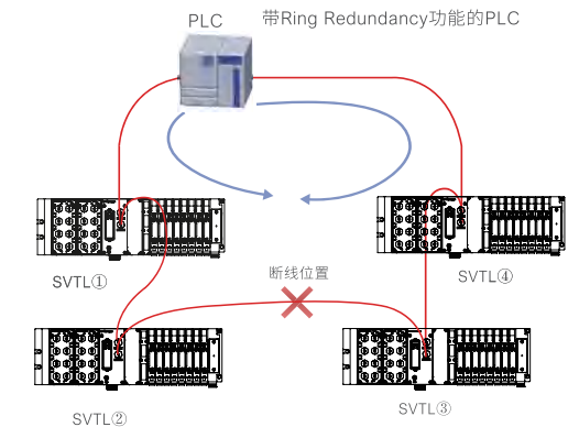
通信电缆断路时信息的流向
