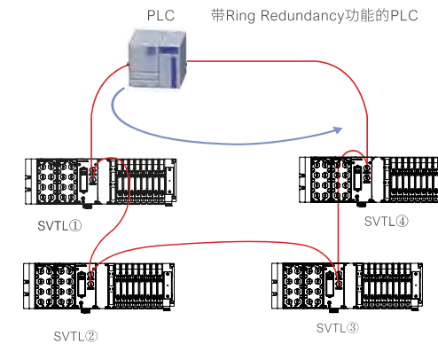
通常状态下信息的流向
